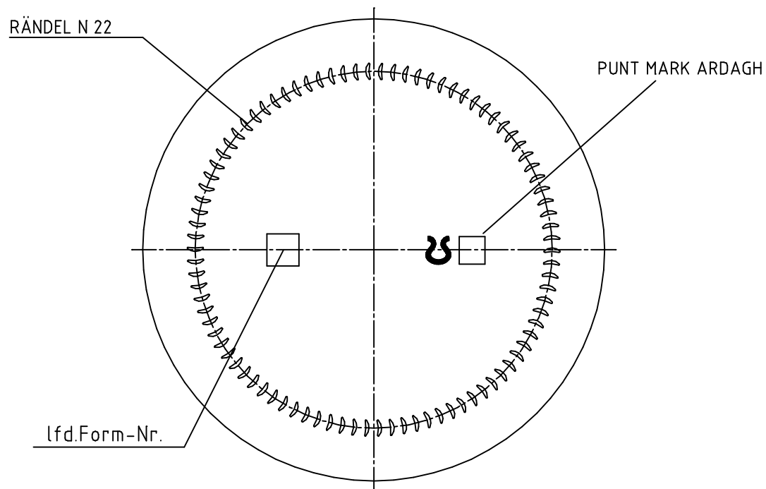
BODENANSICHT
